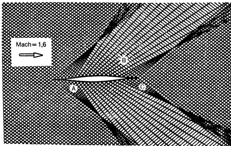
FIG. B.12 – Écoulement supersonique autour d'un profil. Caractéristiques.
