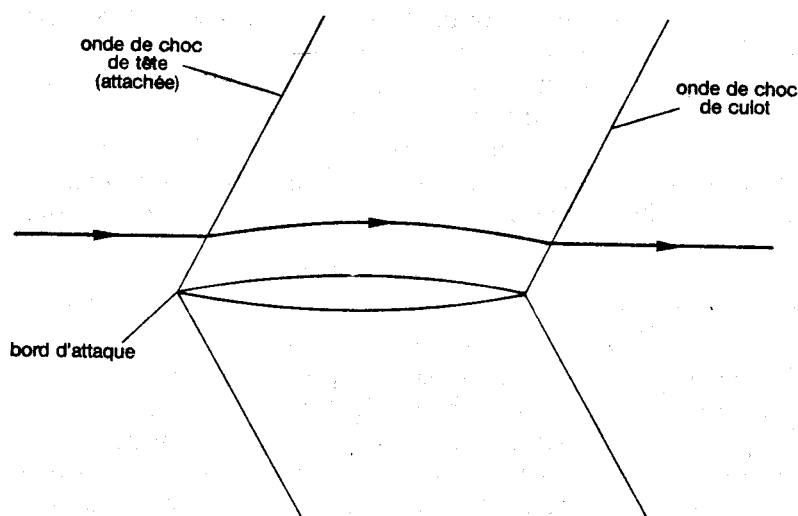
FIG. 5.2 – Ondes de choc autour d'un profil d'aile mince.
