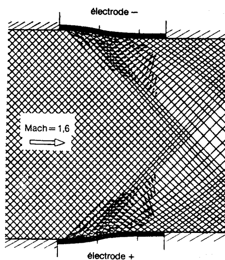
FIG. B.11 – Écoulement supersonique dans un convergent, sans onde de choc.
