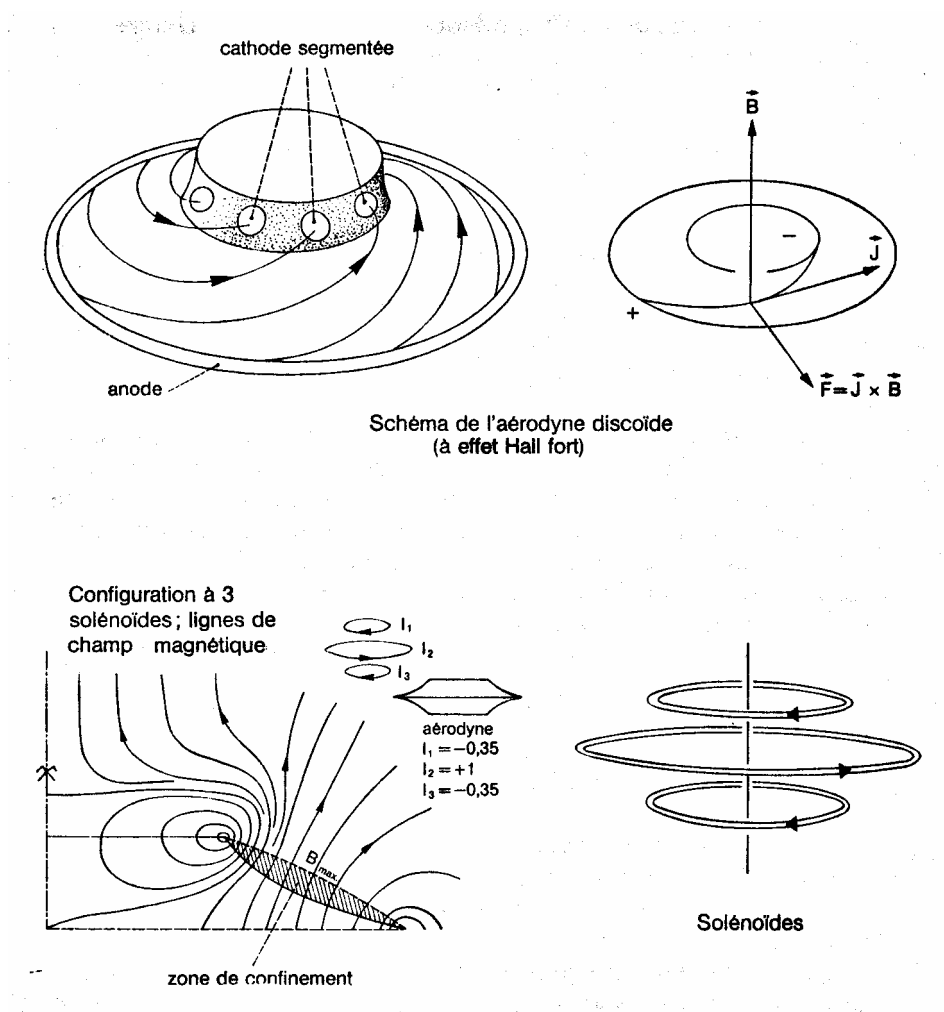
FIG. 2.1 – La géométrie magnétique de l'aérodyne MHD discoïde. Confinement pariétal.
