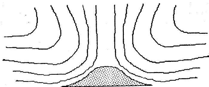
FIG. D.7 – Écoulement MHD produit par un aérodyne MHD discoïde au voisinage du sol, puis loin du sol.
