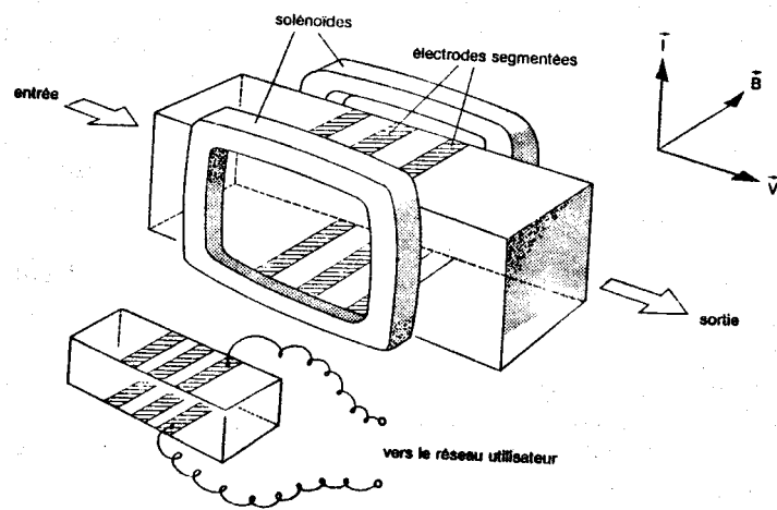
FIG. A.2 – Générateur MHD.
