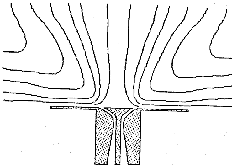
FIG. D.6 – Schéma de l'écoulement induit par un jet radial supersonique.
