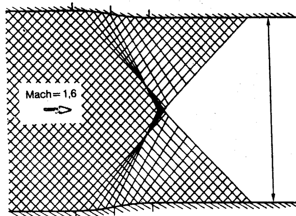
Représentation schématique de la tuyère convergente d'un tube à choc. Le réseau de caractéristiques concourantes indique la présence d'une onde de choc.
