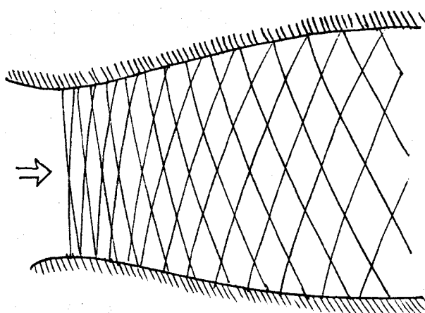
FIG. B.7 – Caractéristiques dans une tuyère divergente.
