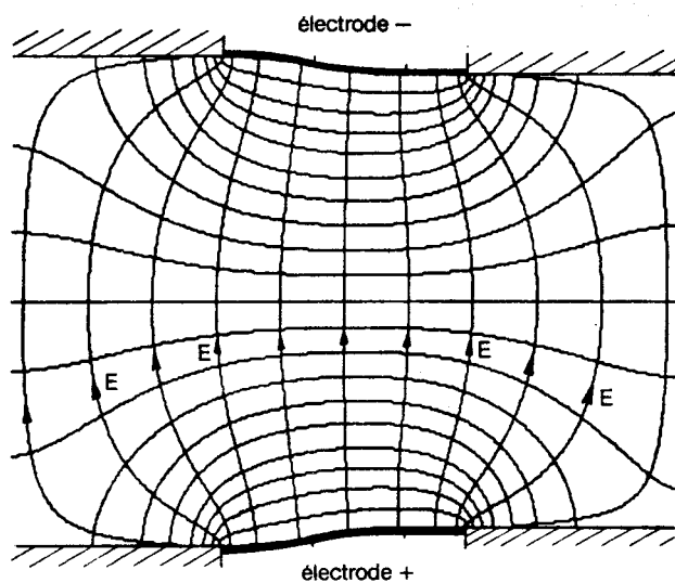
FIG. B.10 – Distribution du courant électrique dans la veine. Champ magnétique perpendiculaire au plan de figure.
