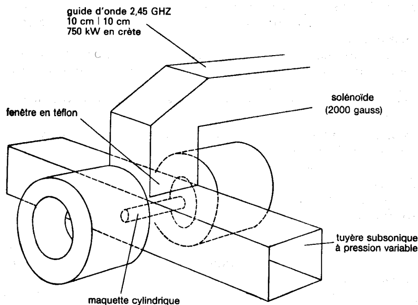
FIG. 5.1 – Schéma de l'expérience du groupe d'étude.
