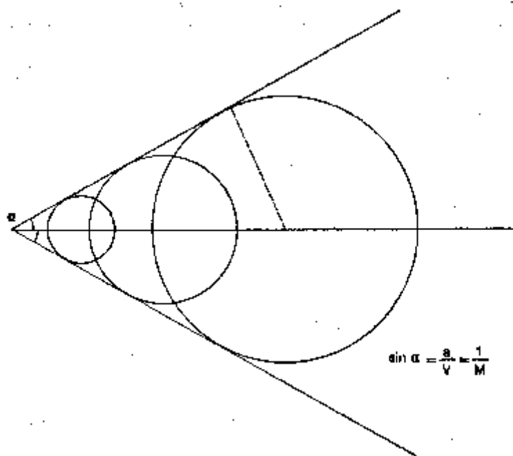
FIG. B.6 – L'Angle de Mach.
