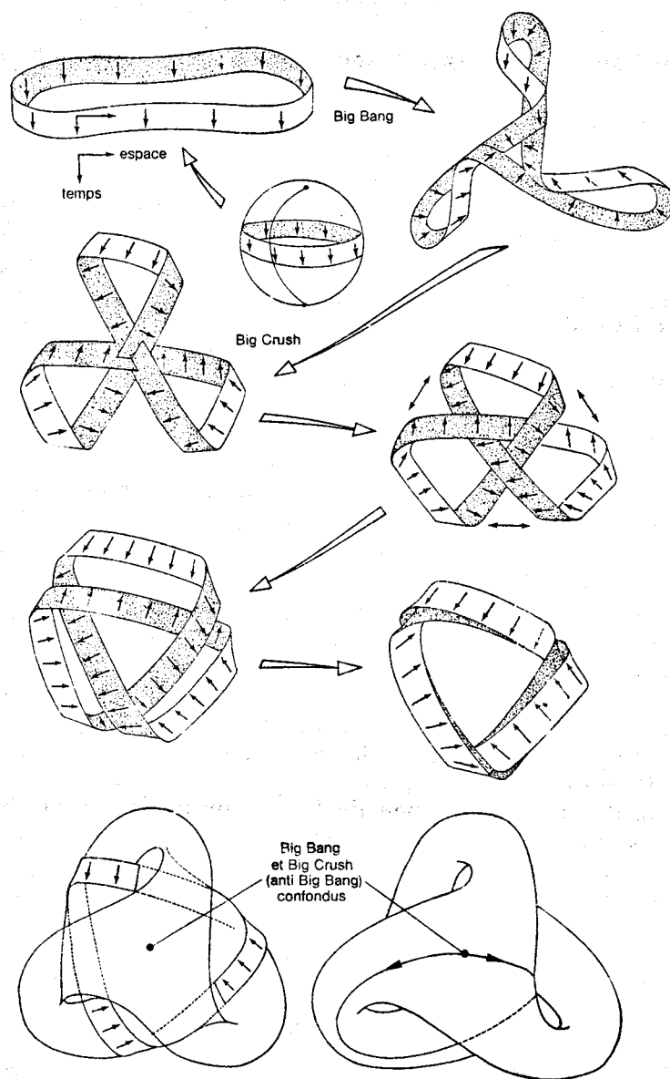
FIG. C.8 – À partir d'une image bidimensionnelle du modèle d'espace-temps de Friedman (sphère) où les pôles figurent le Big Bang et l'anti Big Bang, création des feuillets gémeaux d'espace-temps, avec mise en opposition des flèches du temps. La sphère se transforme en revêtement à deux feuillets de la surface de Boy.
