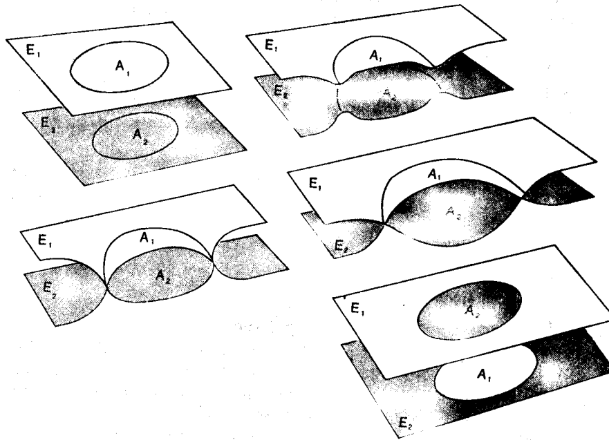
FIG. C.9 – Échange de domaines entre deux espaces jumeaux.
