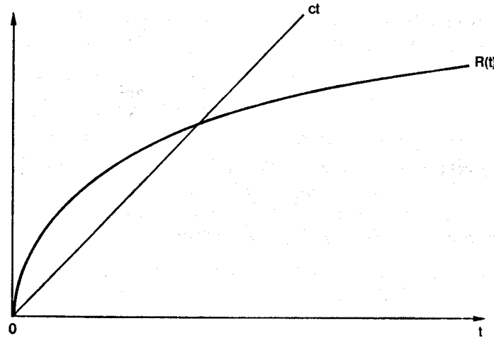
FIG. C.2 – Comparaison entre la distance moyenne inter-particulaire R et « l'horizon cosmologique » ct .
