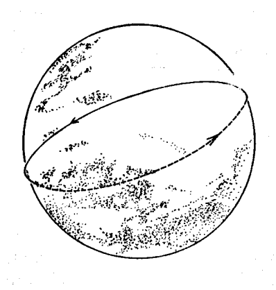
FIG. C.1 – Géodésique de la sphère.
