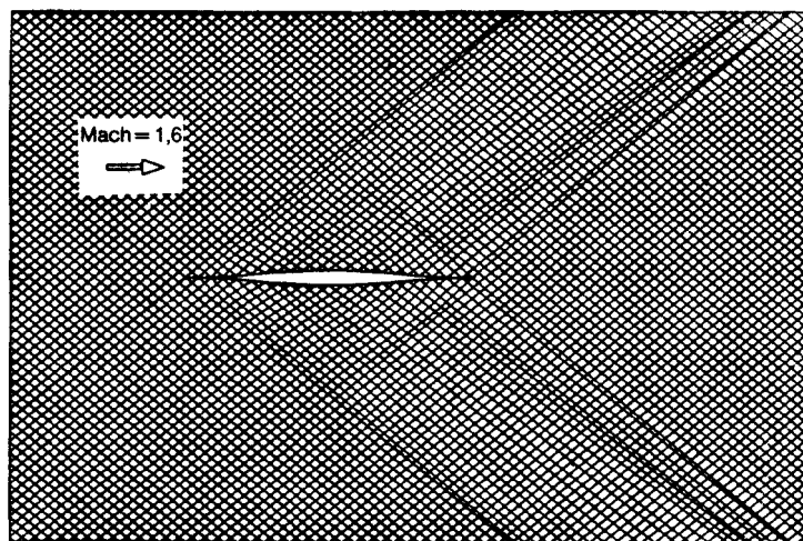
FIG. B.13 – Annihilation des ondes de choc autour d'un profil mince. Nombre de Mach : 1,6.
