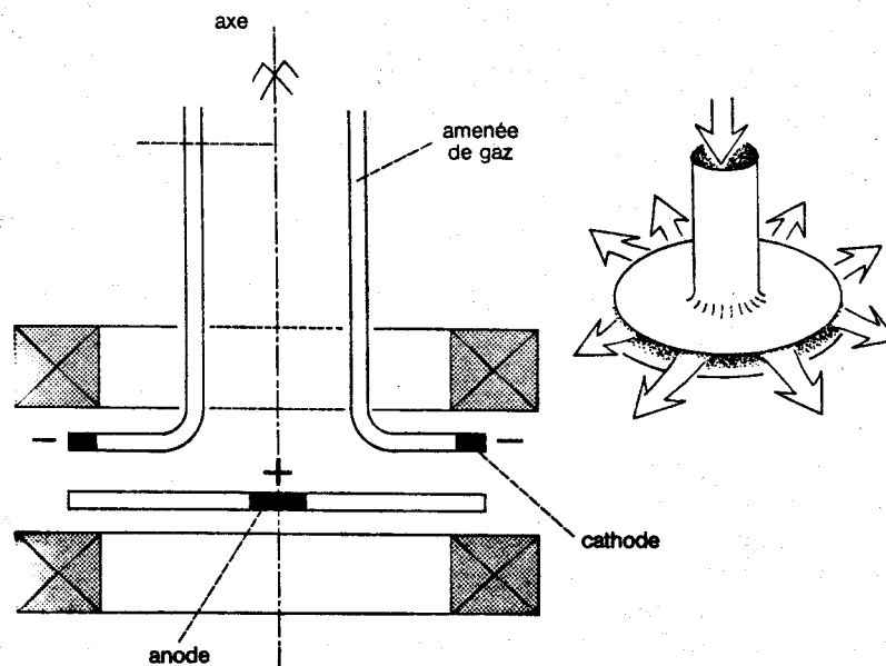
FIG. B.5 – Tuyère-disque.
