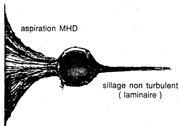
FIG. 3.2 – Écoulement MHD autour d'un cylindre (1976). Noter l'effet d'aspiration sur la partie frontale, à gauche, et l'absence de turbulence de sillage, sur la droite.
