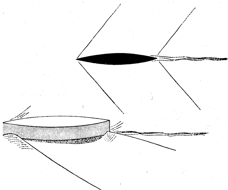
FIG. B.2 – Ondes de choc apparaissant autour d'un profil d'aile biconvexe ou des vagues d'étrave et de poupe d'un navire.
