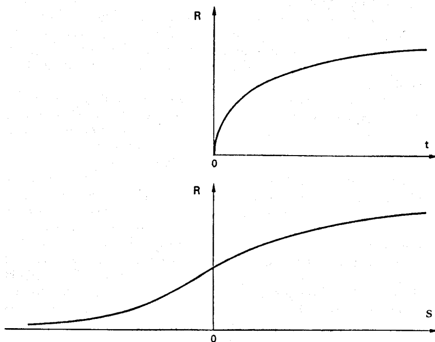
FIG. C.3 – Espace-temps ou espace-entropie.
