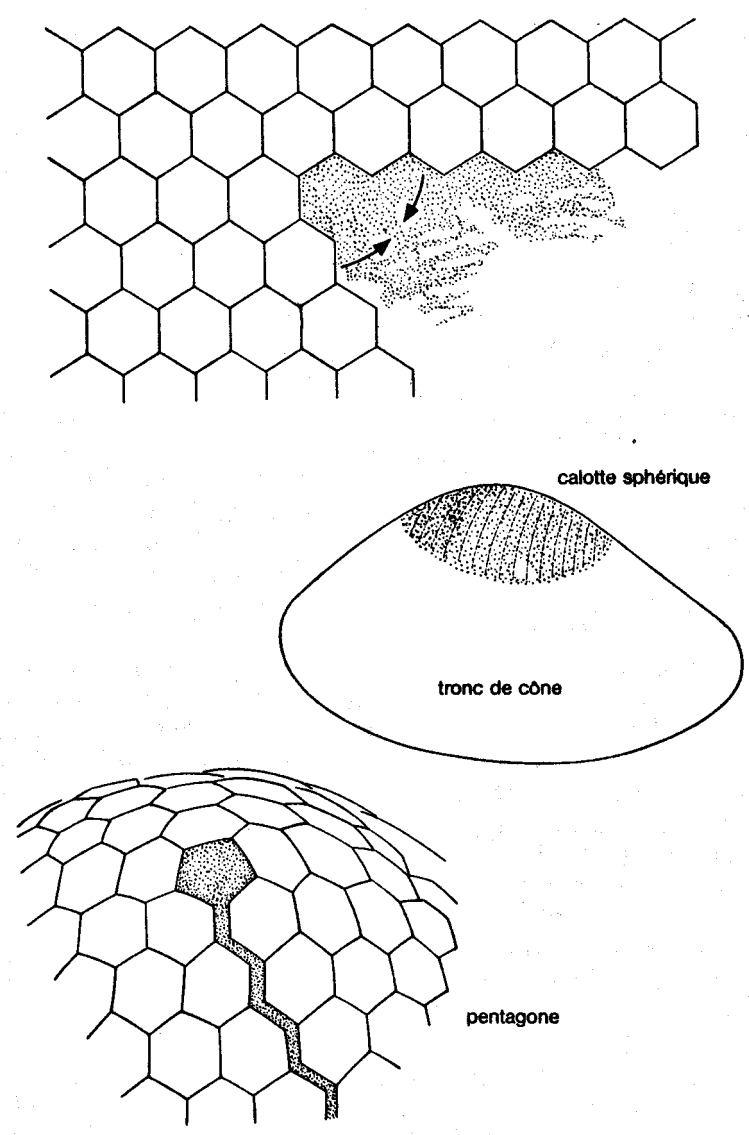
FIG. C.7 – Pavage avec des éléments différents. Recollement de métriques.
