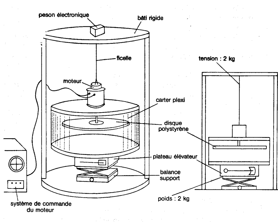
FIG. 3.1 – La machine à antigravitation.
